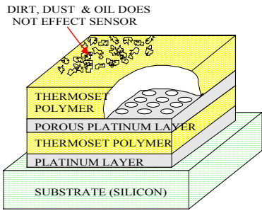
热固聚酯电容式湿度传感器结构
